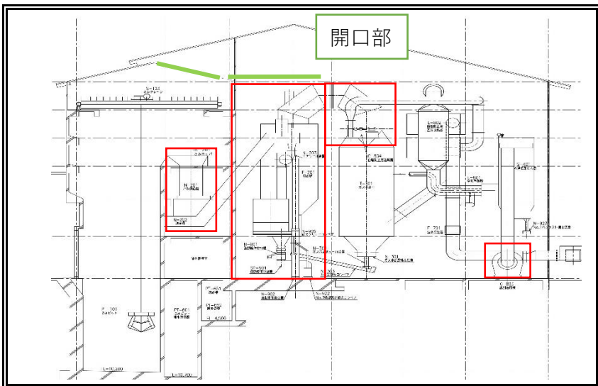
機器配置断面図
