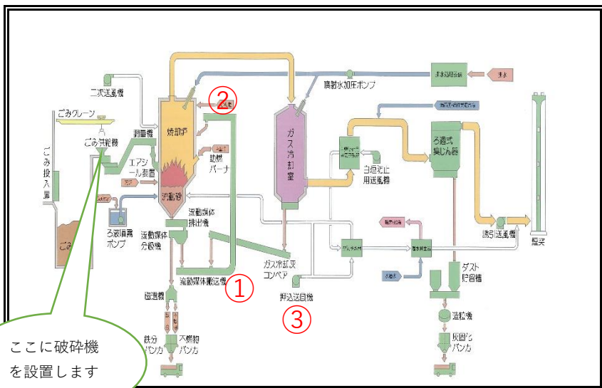
ごみ破砕機図
