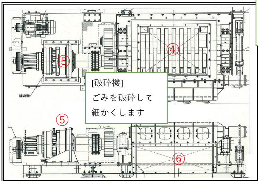
ごみ破砕機図
