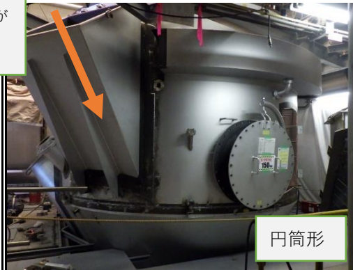
白煙防止用送風機サイレンサー④
