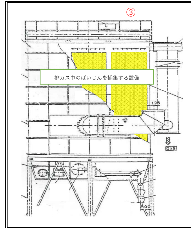
ろ過式集じん器部分補修 ろ過式集じん器図面（立面図）
