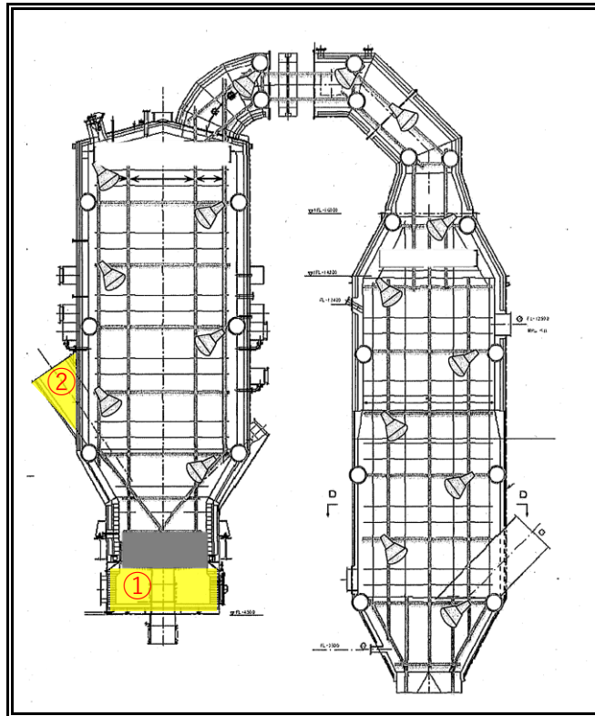
焼却炉・ガス冷却塔耐火工事 耐火施工計画図（立面図）
