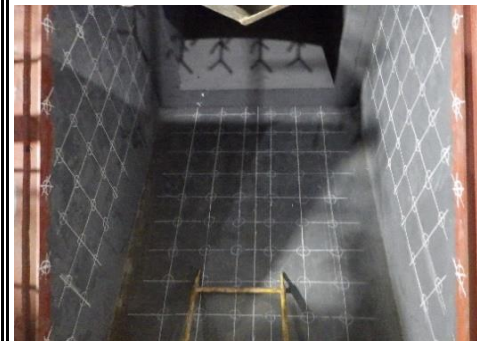
給じん口耐火施工②
