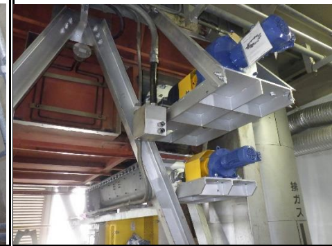
ろ過式集じん器 バグフィルタスクリーン等据付
